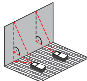
Пифагор 2 варианта
